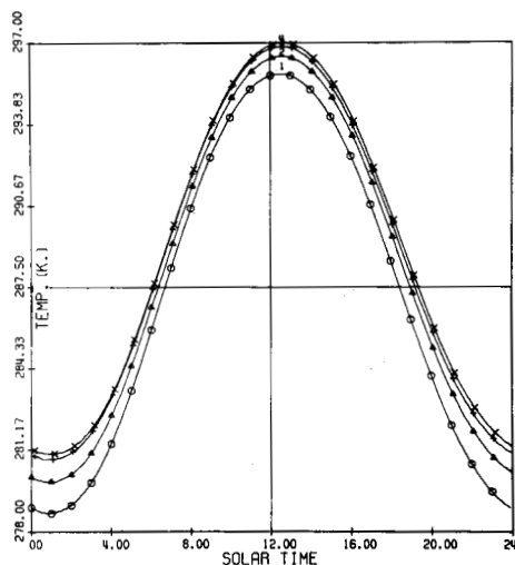
FIG. 1. Surface thermal response; stratigraphy: 10 cm. wet peat above sandy gravel; 1) Active layer depth 10 cm.; 2) Active layer depth 20 cm.; 3) Active layer depth 30 cm.; 4) Active layer depth 40 cm.
